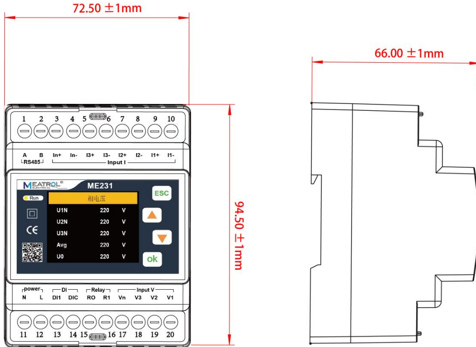
电表尺寸图
