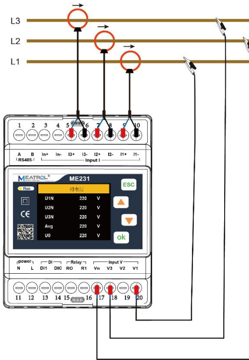
三相三线 3CT
