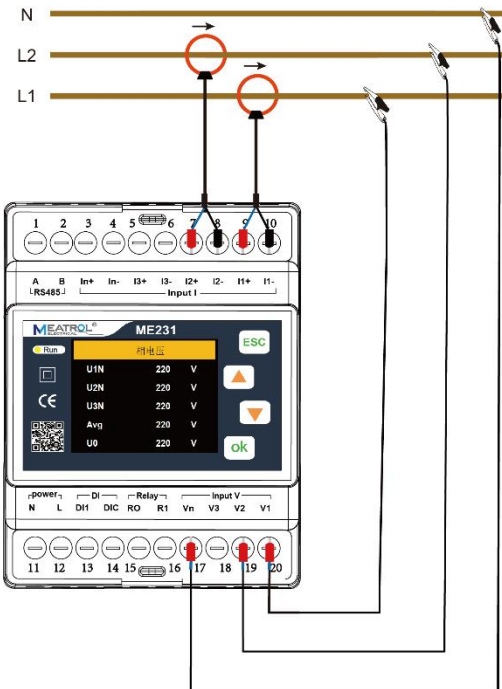
一相三线
