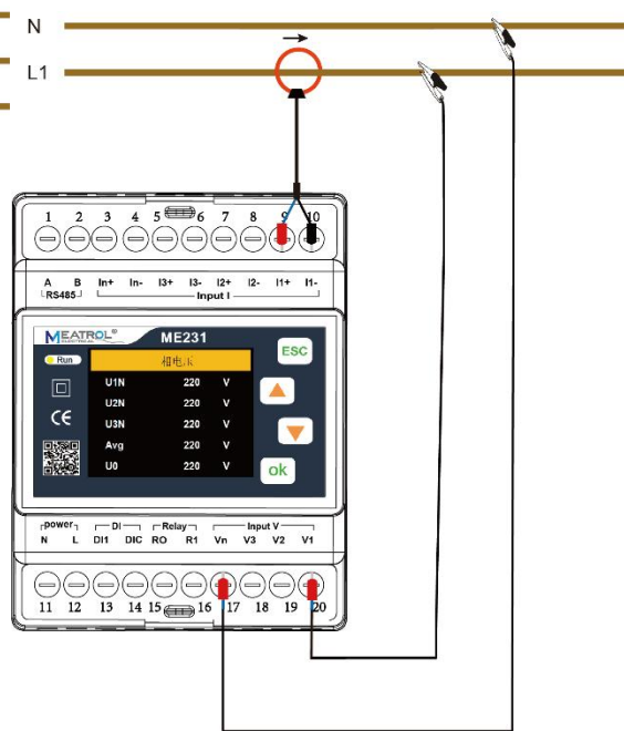
一相两线
