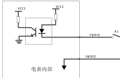
数字输入接口连接示意图
